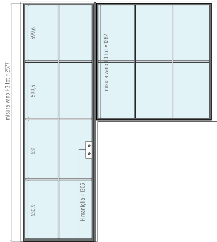
Vista frontale - Vista lato a spingere
