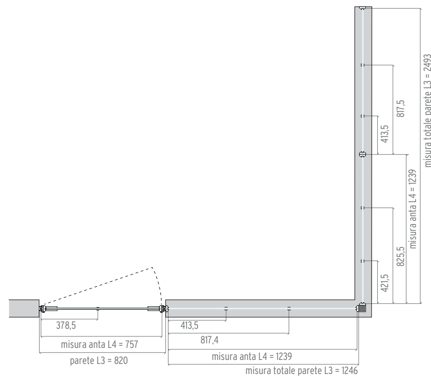
Vista frontale - Vista lato a spingere
