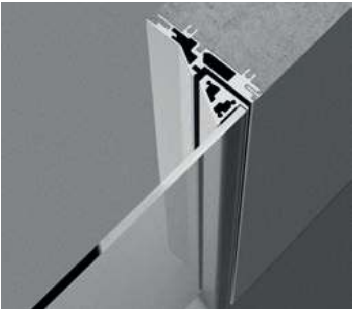
NUOVO PROFILO BLADE. Telaio murato per un effetto Filomuro. Assenza di mostrine. NEW BLADE PROFILE. Frame built into wall for a Filomuro effect. No trim. NOUVEAU PROFIL BLADE. Cadre maçonné pour un effet Filomuro. Sans couvre-joints NUEVO PERFIL BLADE. Marco empotrado efecto a ras de pared. Ausencia de tapajuntas. NEUES BLADE PROFIL. Eingemauerte Zarge für Filomuro-Effekt. Ohne Blendrahmen. НОВЫЙ ПРОФИЛЬ BLADE. Косяк, встроенный в стену для эффекта Filomuro (вровень в стену). Отсутствие накладок.
